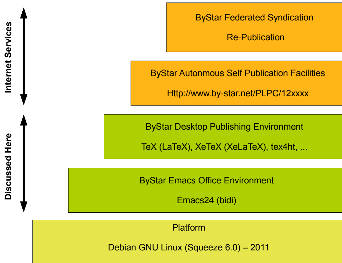
شکل ۱ : publicationLayers
